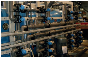
Meriveden esisuodatinlaitteistoa
